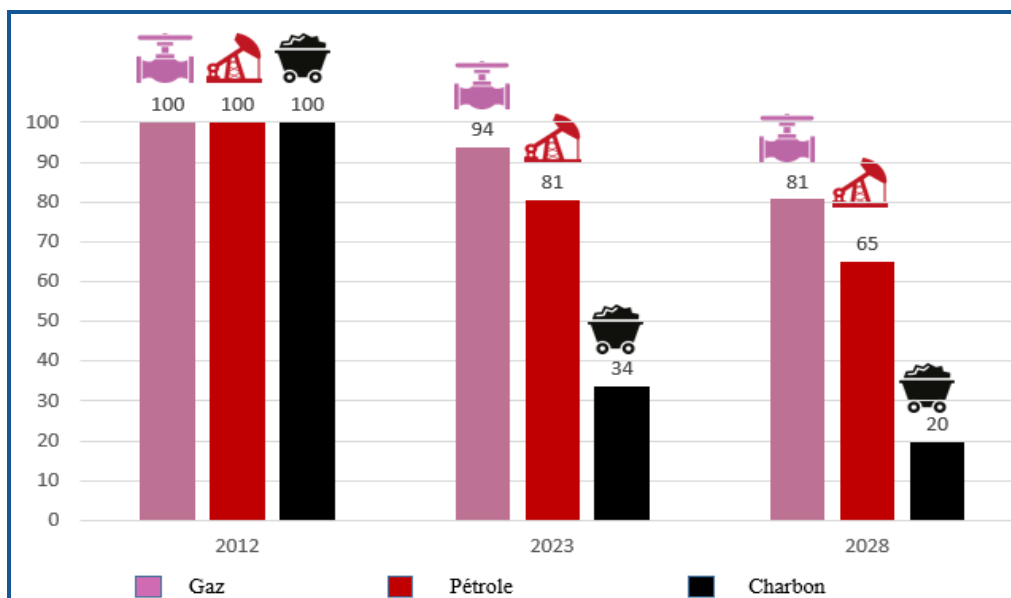
Figure 2 : Réduction de la consommation primaire d'énergie fossile par vecteur énergétique
